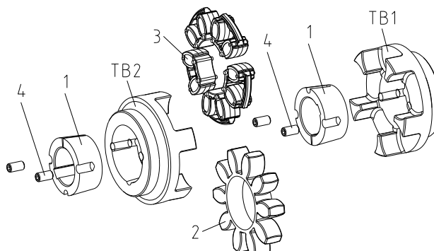
Рис. 8: ROTEX® Исполнение с Тарег-зажимной втулкой
