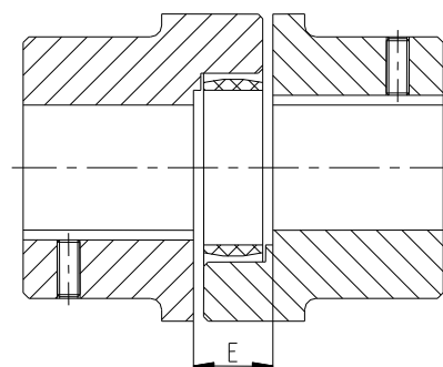
Рис. 11: Монтаж муфты
