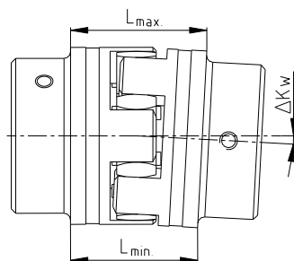
Угловые смещения
