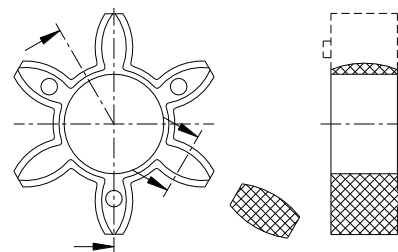
Рис. 17.2: ROTEX®- зубчатый венец
