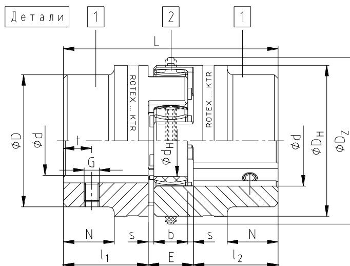
Рис. 3: ROTEX® (материал: сталь)
