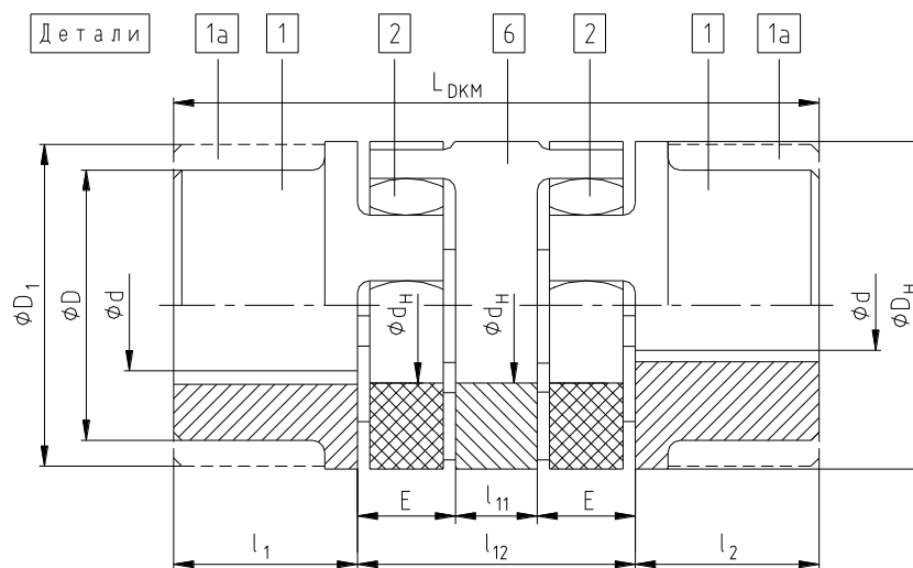
Рис. 4: ROTEX® исполнение DKM
