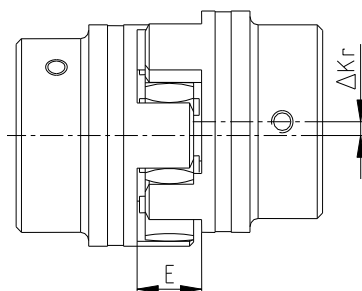
Радиальные смещения
