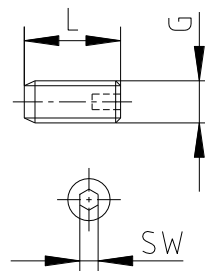
Рис. 13: Withworth-установочный винт (BSW)
