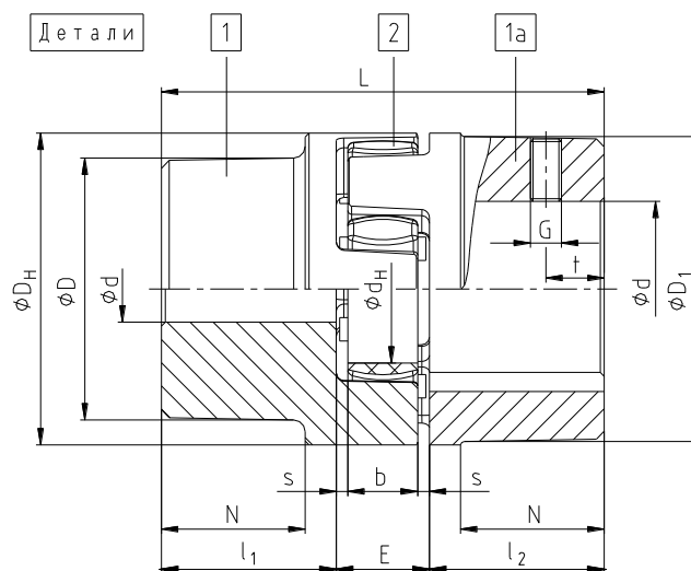
Рис. 1: ROTEX® (Материал: спечённая порошковая сталь, алюминий литой под давлением (Al-D) и алюминий (Al-H))
