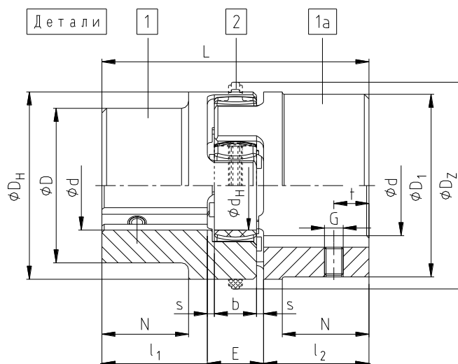
Рис. 2: ROTEX® (материал: GJL/GJS)
