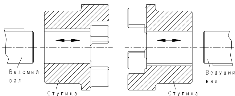
Рис. 10: Монтаж ступиц
