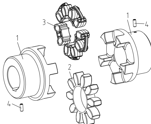
Рис. 6: ROTEX®
