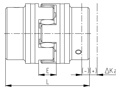
Осевые смещения
