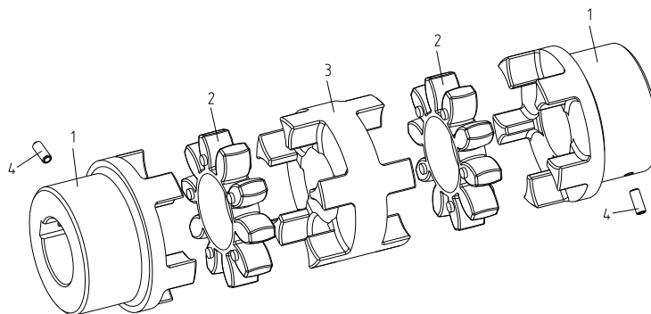
Рис. 7: ROTEX® исполнение DKM
