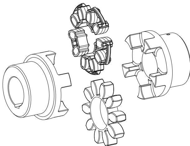
Рис. 16: ROTEX®-муфта
