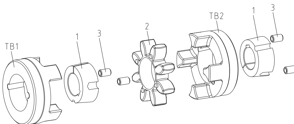
rysunek 8: ROTEX® wykonanie do zbieżnej tulei zaciskowej
