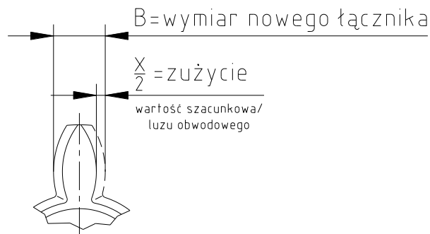
rysunek 24: zużycie łącznika
