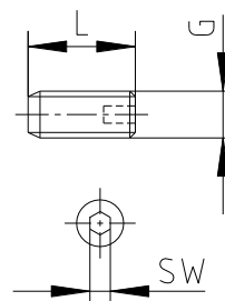
rysunek 18: wkręt mocujący (BSW)
