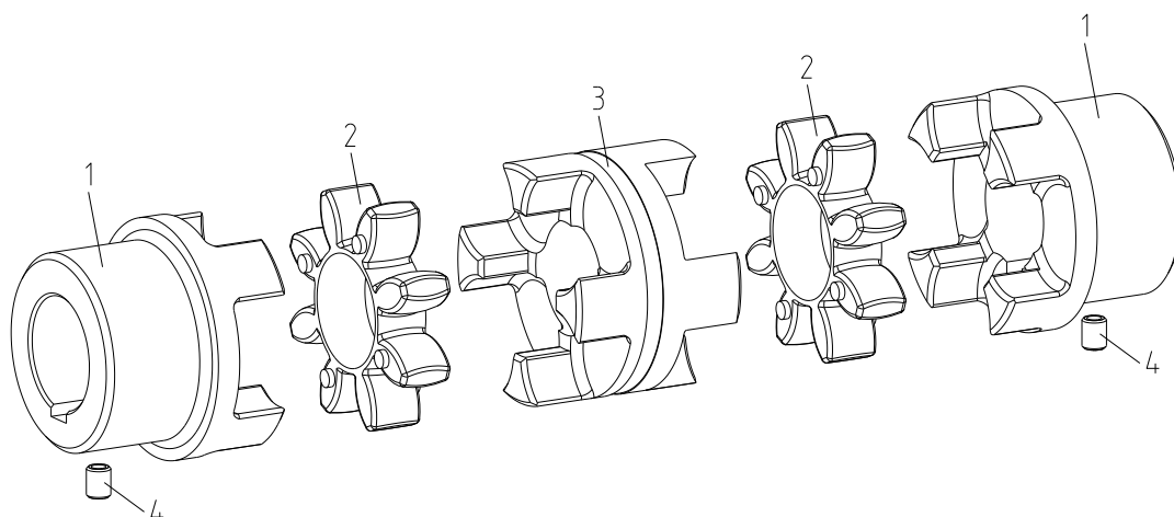
rysunek 7: ROTEX® wykonanie DKM
