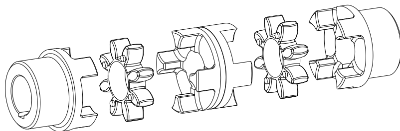
Type nr. 018 - DKM dobbelbåndkløber
