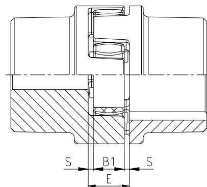
Fig. 12: Koblingsmontage
