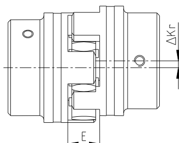
Radialforskydninger
