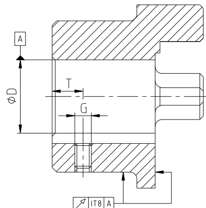
Fig. 9: Rund- og planløbsnøjagtighed
