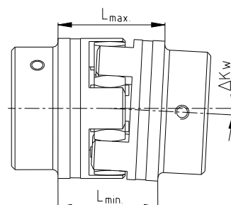
Vinkelforskydninger
