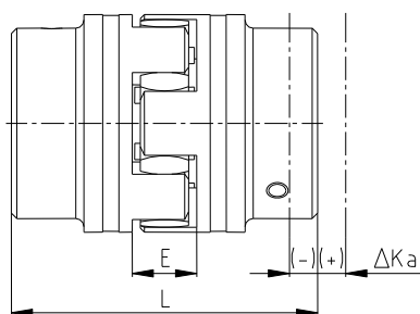
Aksialforskydninger
