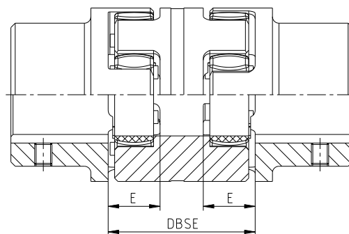
Fig. 16: Koblingsmontage
