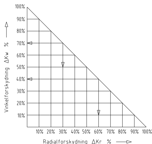
Fig. 20: Forskydningskombinationer
