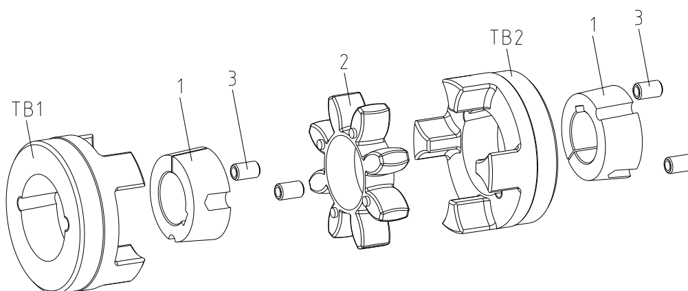
Fig. 8: ROTEX® type med Taper-spændebøsning
