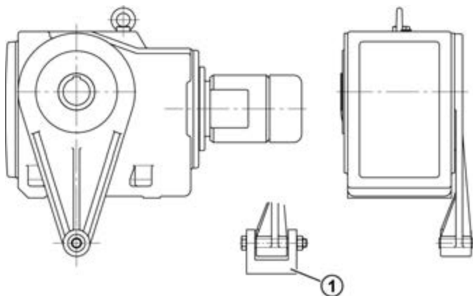
Figure 13: Fixation du bras de réaction sur les réducteurs à couples coniques et à vis sans fin
