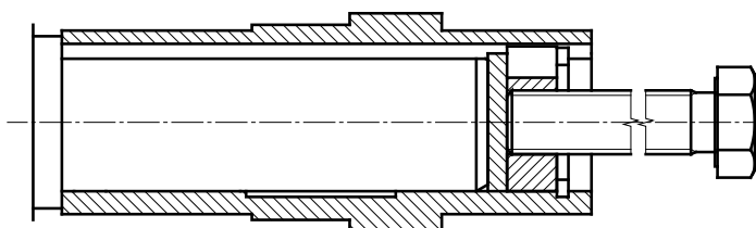
Figure 11: Démontage à l'aide d'un dispositif de démontage
