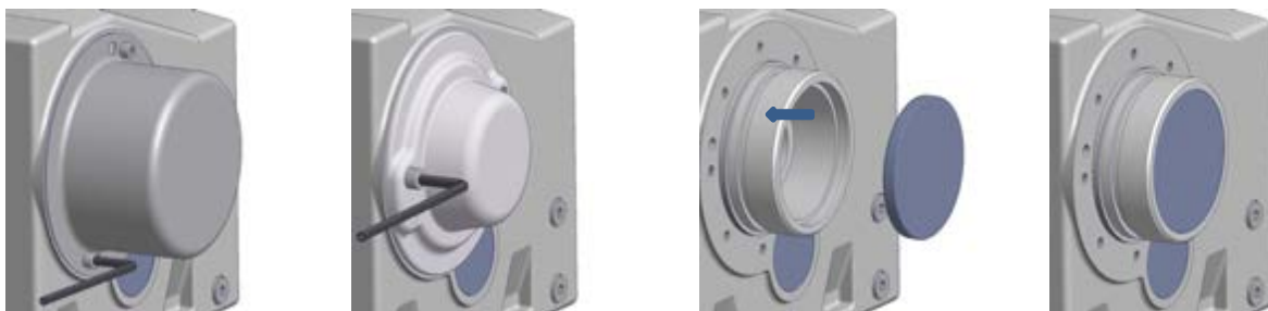
Figure 15: Montage du capot de protection option SH, option H et option H66
