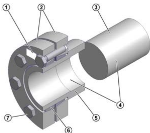
Figure 14: Arbre creux avec frette de serrage
