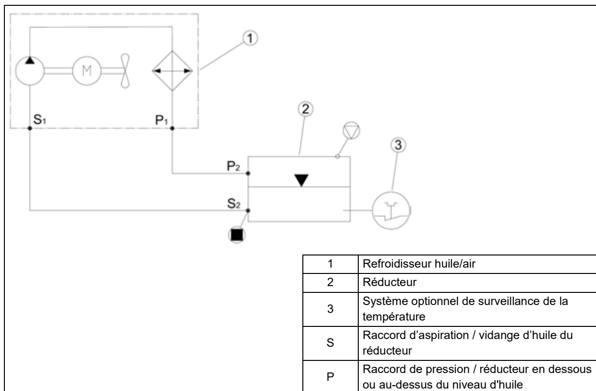
Figure 19: Raccordement de l'installation de refroidissement
