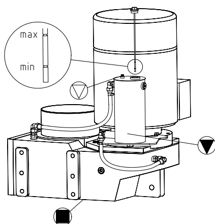
Figure 25 : Vérification du niveau d'huile avec réservoir de niveau d'huile
