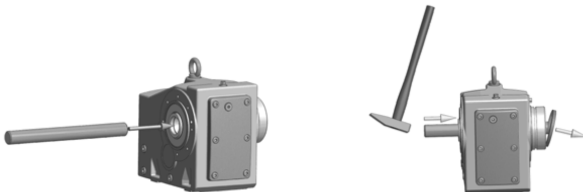
Figure 8: Démontage du bouchon de fermeture monté en usine
