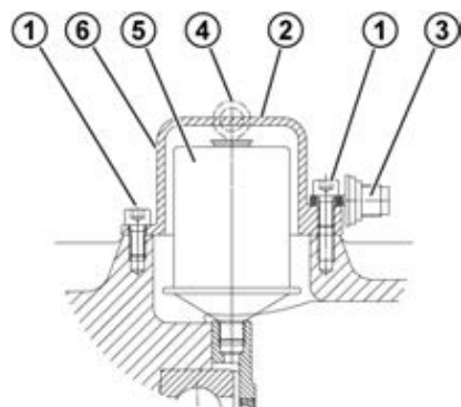
Figure 21: Activation du graisseur automatique dans le cas d'un montage de moteur standard
