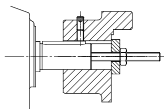
Figure 5: Exemple d'un dispositif de montage simple
